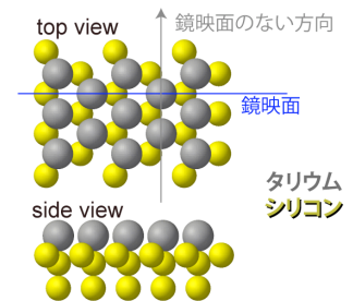
図3 タリウム吸着シリコン表面
