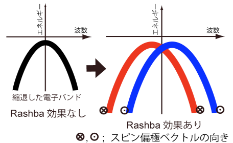
図2 ラシュバ効果による電子バンドの分裂
