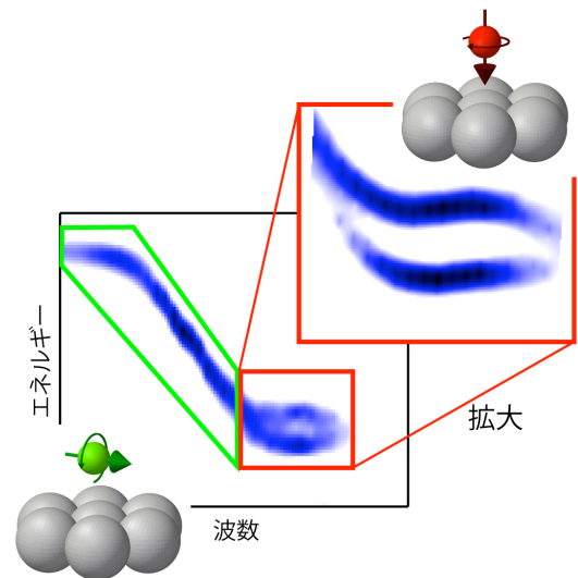
図4 タリウム吸着シリコン表面の電子バンド。
